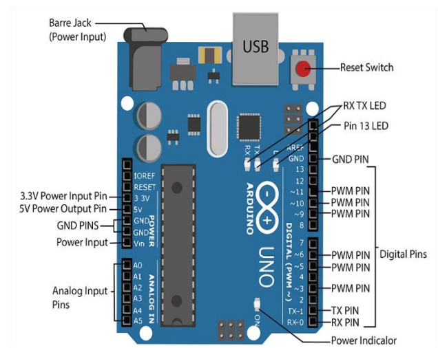
Fig. 1. Diagram of Arduino Uno.
