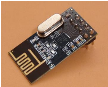
Fig 3.9 RF Module
