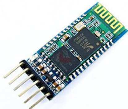
Fig 3.8 Bluetooth Module
